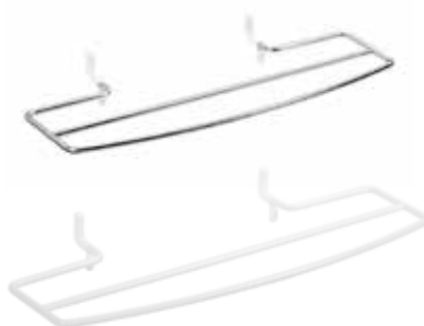
Držák ručníků na otopné těleso (600 × 80 × 220 mm)
