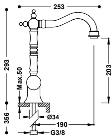
Miscelatore monocomando con leva laterale per lavabo
