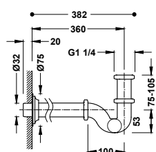
Sifone telescopico con piletta per lavabo
