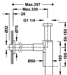
Sifone telescopico rotondo ispezionabile con calotta per lavabo
