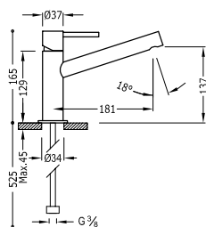
Miscelatore monocomando per lavabo
