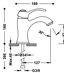
Miscelatore monocomando per lavabo
