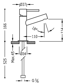
Miscelatore monocomando per lavabo
