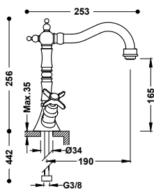
Miscelatore bicomando per lavabo
