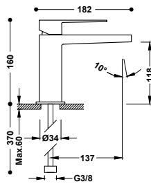
Miscelatore monocomando per lavabo
