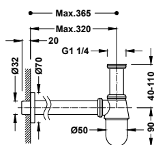
Sifone telescopico a bottiglia ispezionabile con calotta per lavabo
