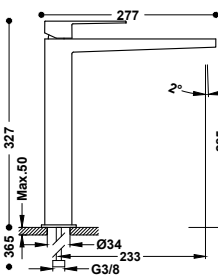
Miscelatore monocomando XXL per lavabo
