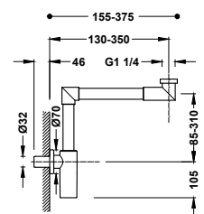
Sifone telescopico a gomito per lavabo
