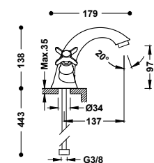
Miscelatore bicomando per lavabo
