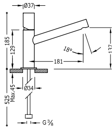
Miscelatore monocomando per lavabo
