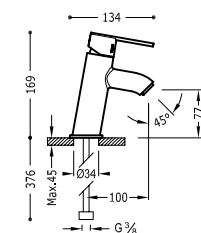
Miscelatore monocomando inclinato per lavabo
