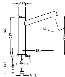
Miscelatore monocomando alto per lavabo
