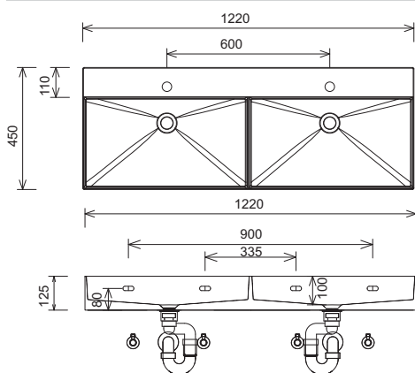
SQUARED WTM 482D / WTO 482D Náčrt otvoru pro výřez armatur
