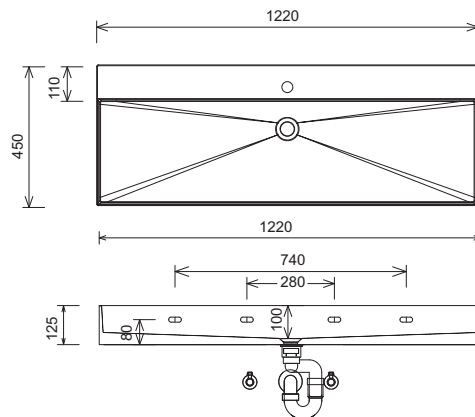
SQUARED WTM 4812 / WTO 4812 Náčrt otvoru pro výřez armatur
