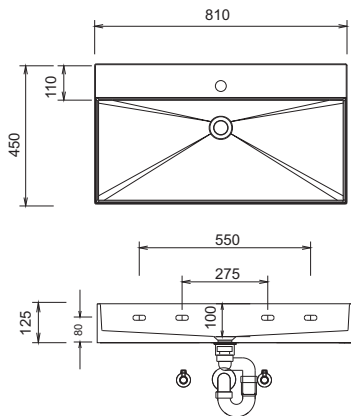
SQUARED WTM 4808 / WTO 4808 Náčrt otvoru pro výřez armatur
