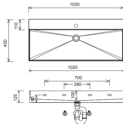
SQUARED WTM 4810 / WTO 4810 Náčrt otvoru pro výřez armatur
