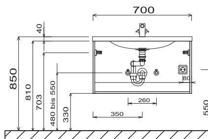
INSTALAČNÍ PŘÍKLADY SET VU70
