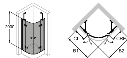
Rohový vstup
