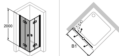
Upevnění vlevo
