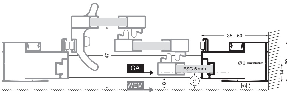
SLIDE triple sliding door
